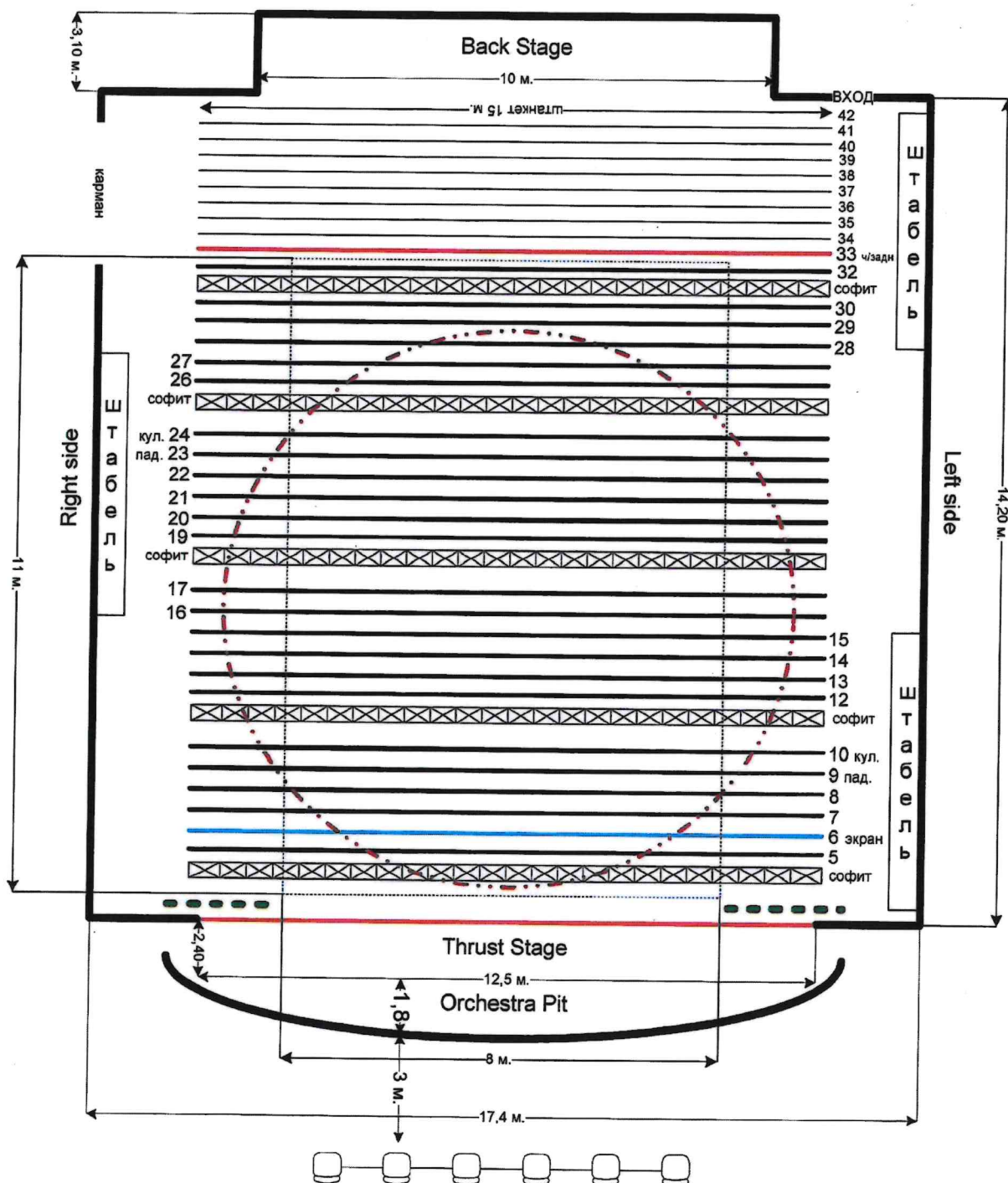
Схема размещения светового оборудования основной сцены МУК ДК «Победа» (пгт Удельная, Раменский МО)
